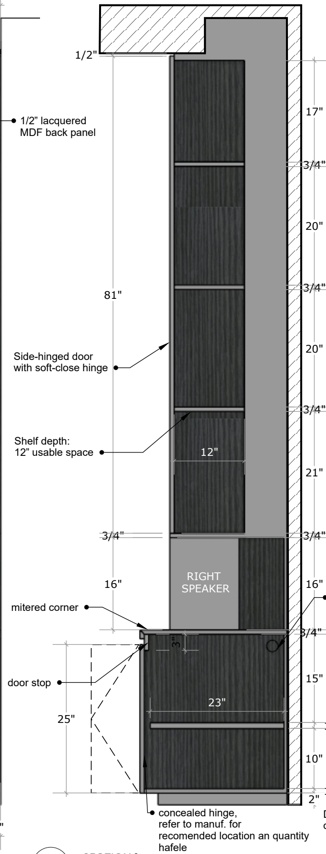
P3 SECTION 1 Scale: 3/4"=1'-0"
