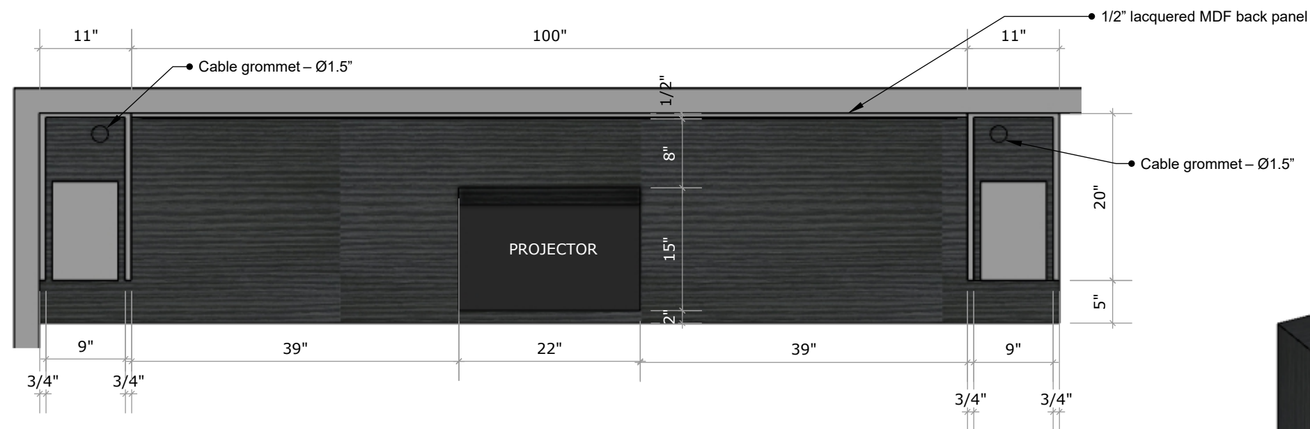
P4 TOP VIEW 1 Scale: 3/4"=1'-0"
