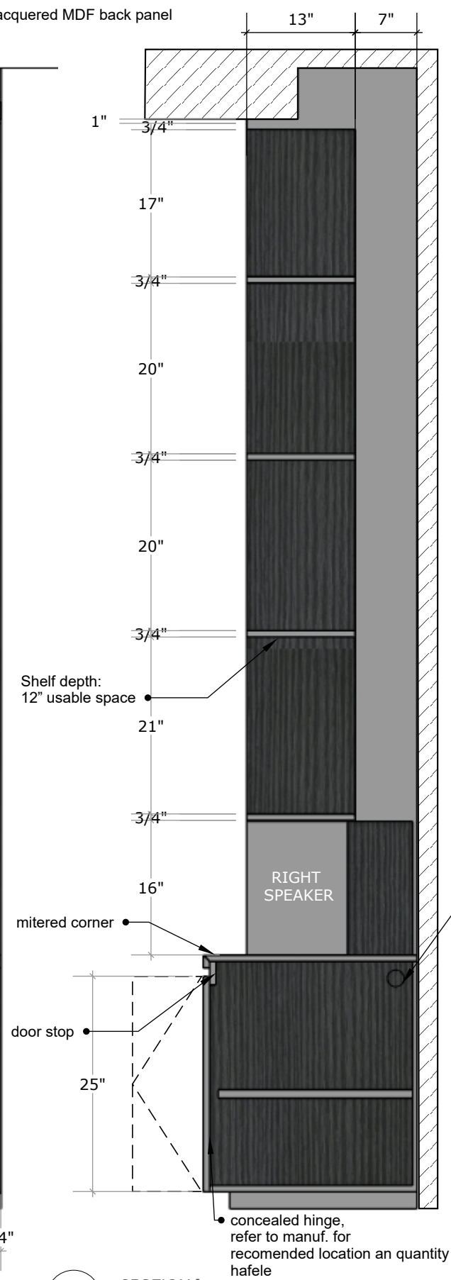
P6 SECTION 1 Scale: 3/4"=1'-0"
