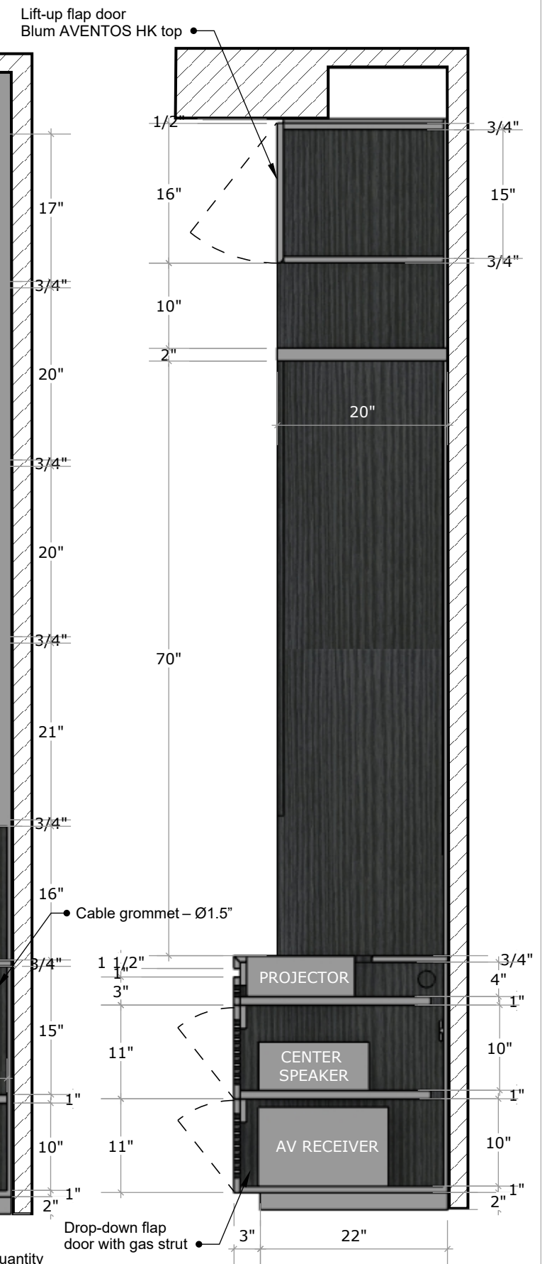
P3 SECTION 2 Scale: 3/4"=1'-0"
