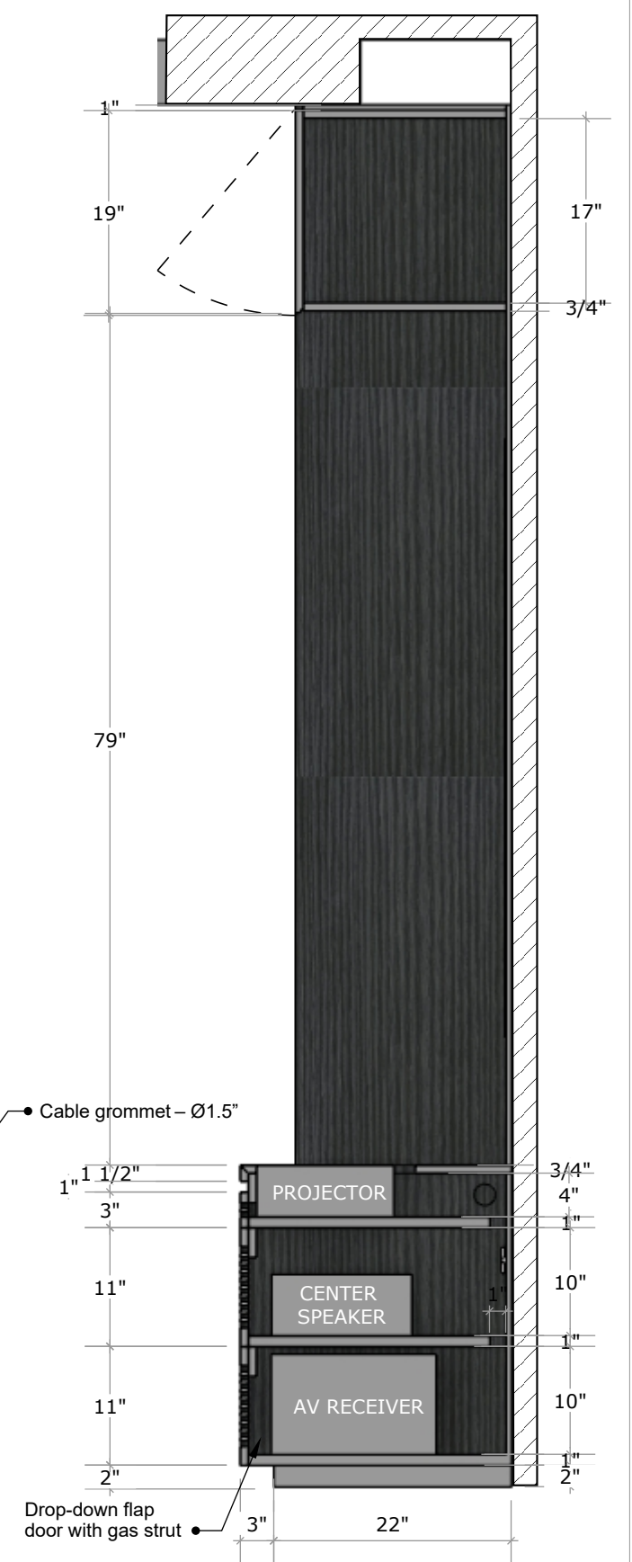
P6 SECTION 2 Scale: 3/4"=1'-0"
