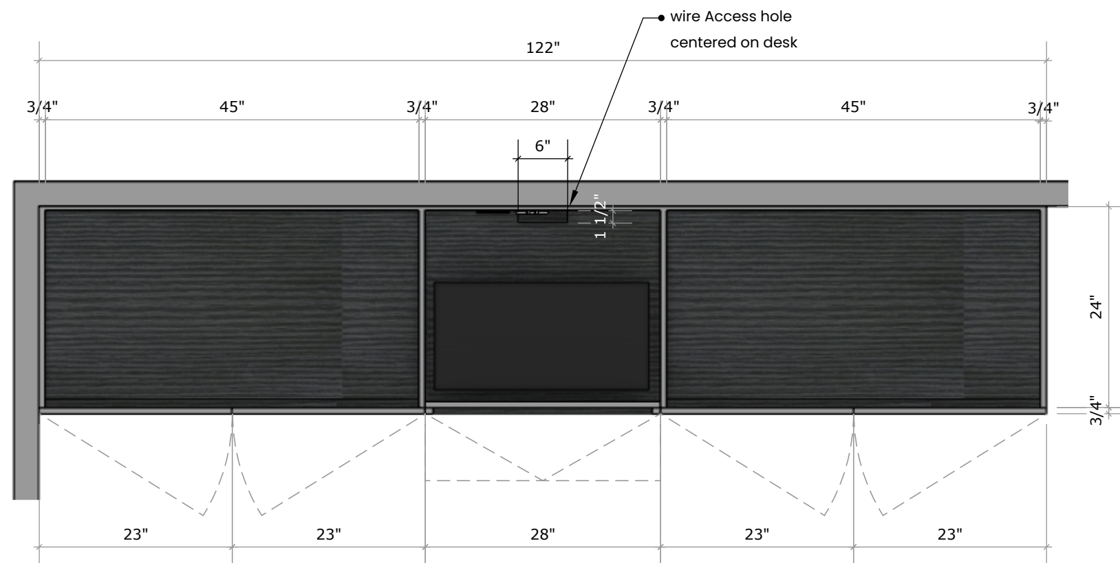
P4 TOP VIEW 2 Scale: 3/4"=1'-0"
